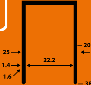
GRAPA 1068 □ 1.4 x 1.6 mm
