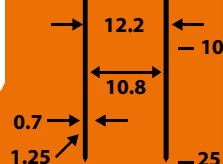
GRAPA 65 □ 0.7 x 1.25 mm
